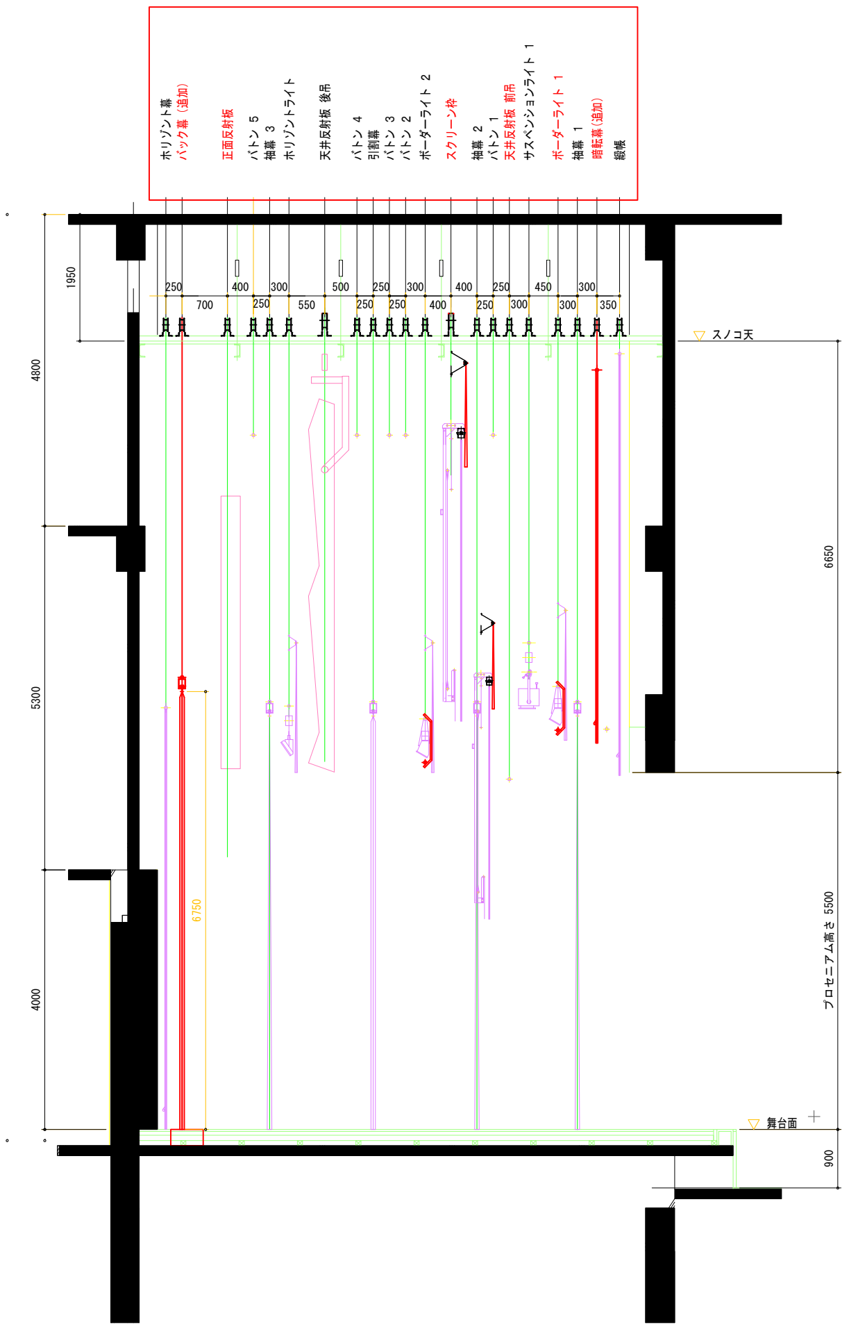
断面図(小ホール)
